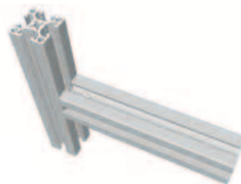
Estado final de unión con conector perpendicular o de cabeza redonda
