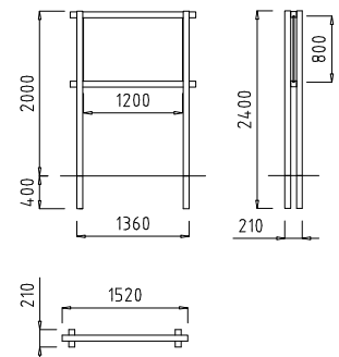
MI013 - MI014 - MI015 E: 1/100
